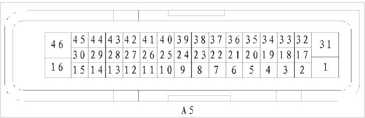
A5：ECU（从进线方向视图）
